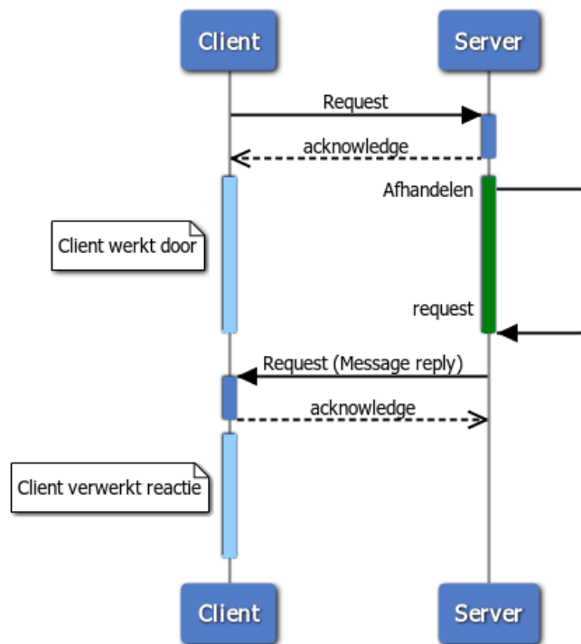
Figuur 10 Asynchroon Request
