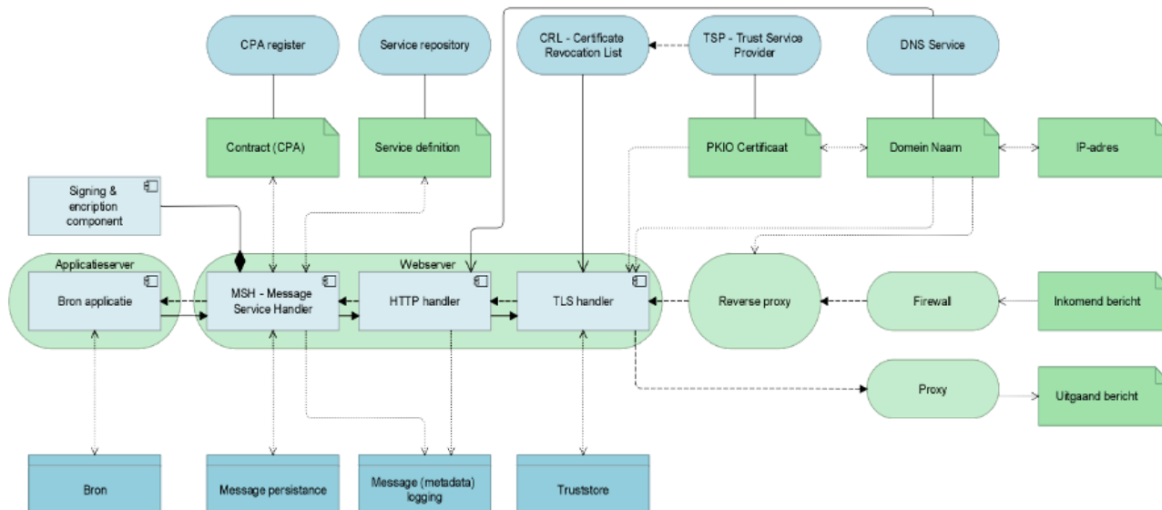
Figuur 9 Referentiemodel gegevensuitwisseling
