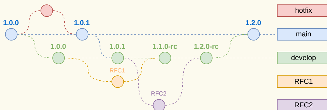
Figuur 7 Gitflow
