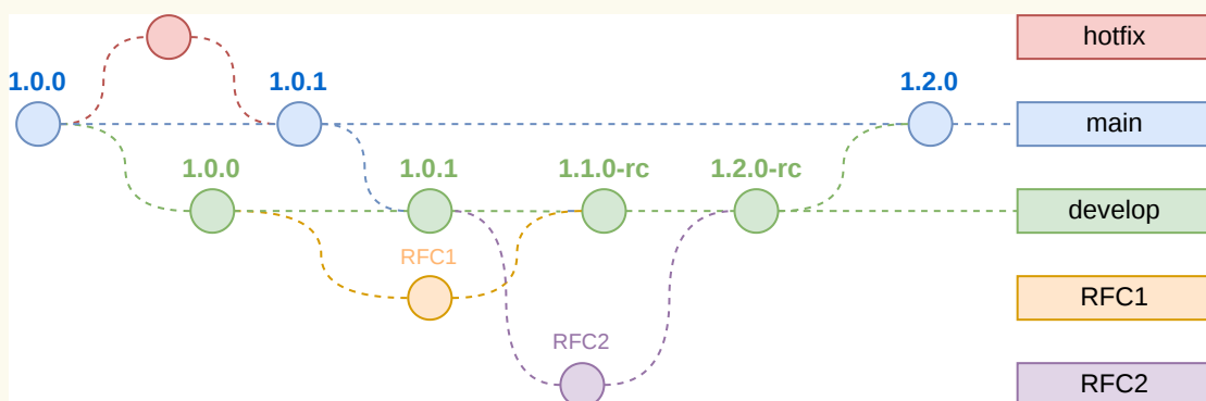
Figuur 5 Gitflow
